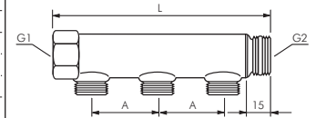
3 Abgänge mit Außengewinde
